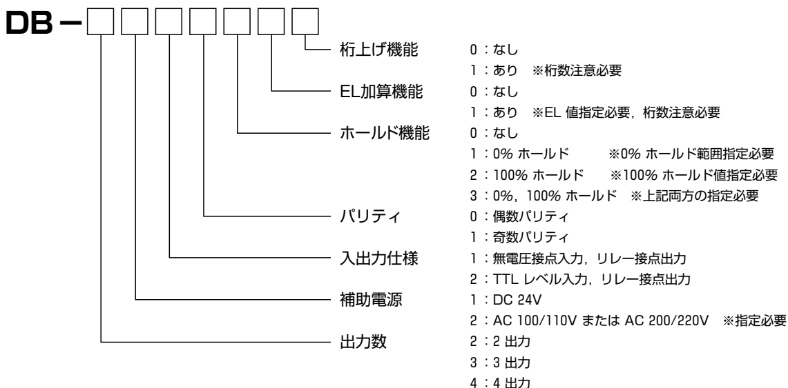
BCD信号分配器
