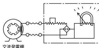
交流発電機 交流発電機で検出する電気式回転計
