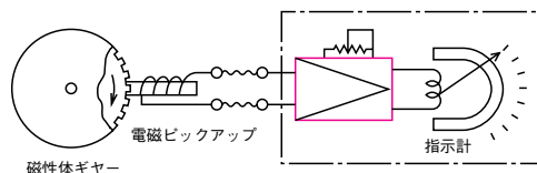
磁性体ギヤ 電磁ピックアップで検出する電気式回転計
