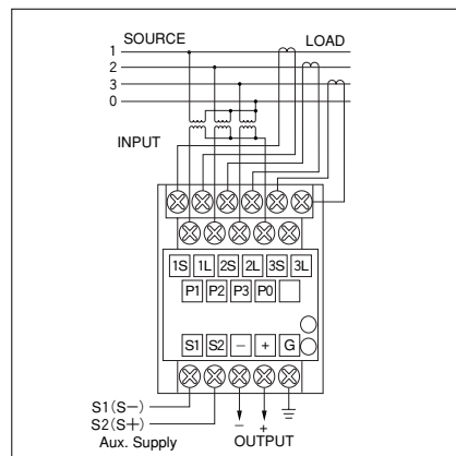
NGM-□4A 三相4線
