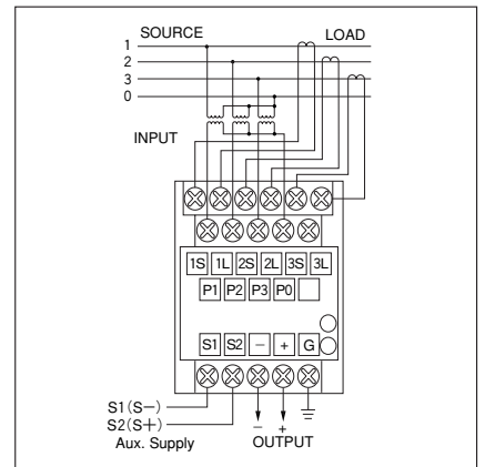
EGM-□4A 三相 4線
