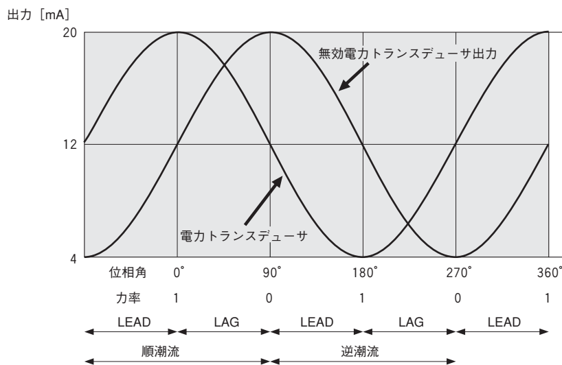
(図4) EGM形、RGM形の入力位相—出力特性 (入力の電圧・電流を定格状態にし、位相差を変化させたときの出力)
