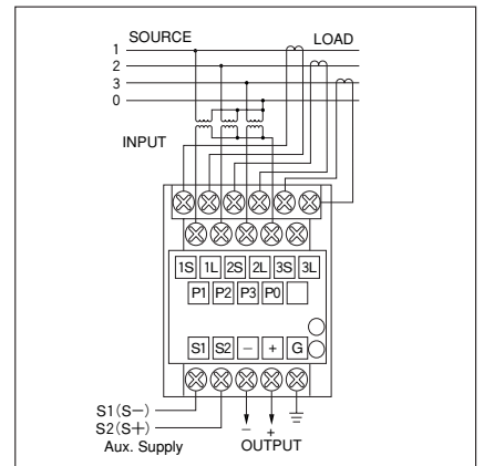
RGM-□4A 三相 4 線
