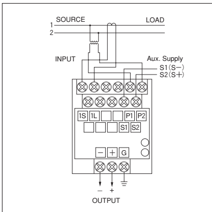
NGM-□1RA 単相 2線
