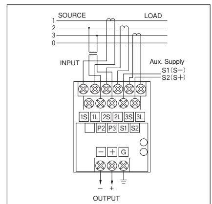
NGM-□4RA 三相 4線
