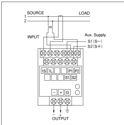
EGM-□1A 単相 2線
