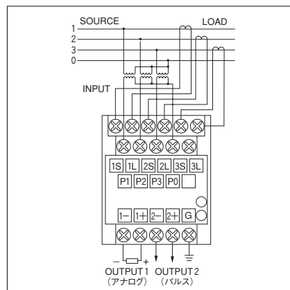
WGM-04A 三相4線
