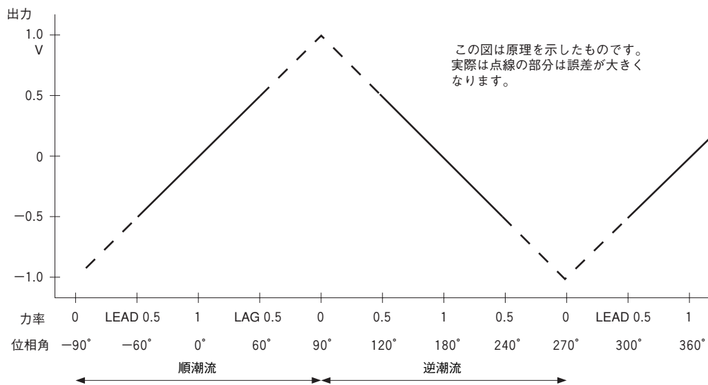
(図5) NGM-R形の入力—出力特性 [入力：LEAD 0.5 ~ 1.0 ~ LAG 0.5] [出力：DC -0.5 ~ 0 ~ +0.5V]
