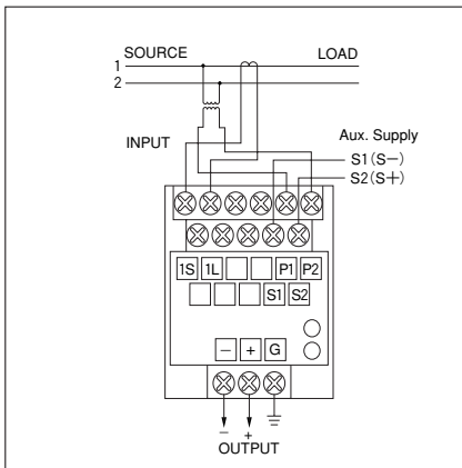
RGM-□1A 単相 2 線
