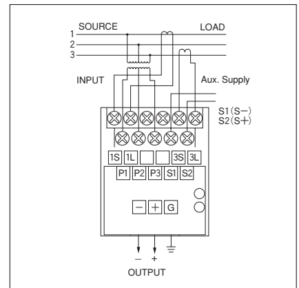
NGM-□3RA 三相 3線
