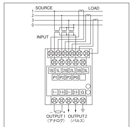
QGM-04A 三相 4 線
